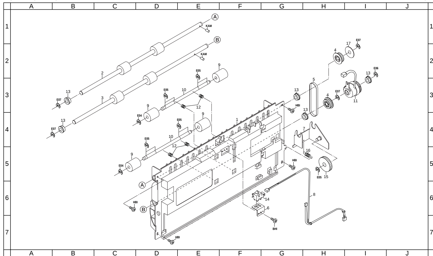
FIG. 1 DUPLEX UNIT
